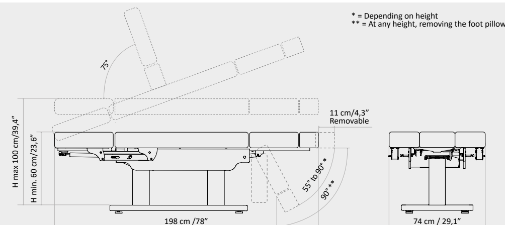
Tilting adjustment / Regolazione basculante
