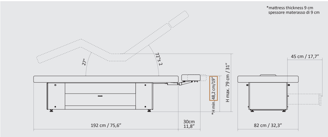
Cabinet base with heated drawer (upon request) Base contenitore con cassetto riscaldato (su richiesta)
